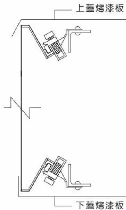
直式、橫式帆布夾具大樣
