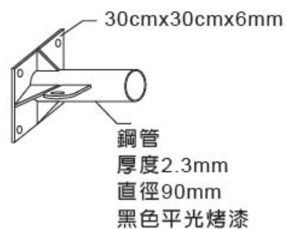
主連接管示意圖
